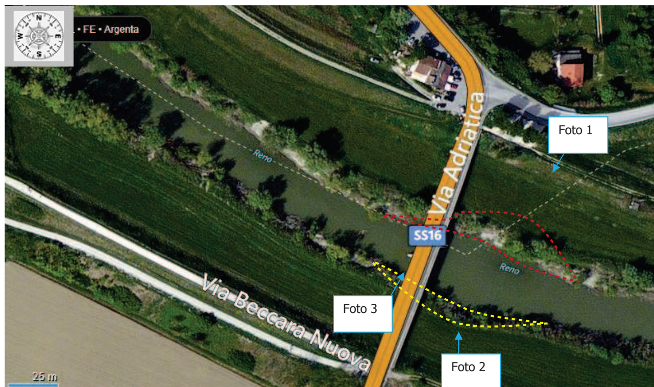
Fig. 8.2 - foto aerea (da Bingmaps 2011) del ponte Bastia (punto critico Ci1). Le aree tratteggiate indicano la dimensione del fenomeno erosivo che interessa le sponde dell'alveo di magra al 31/12/2013.
